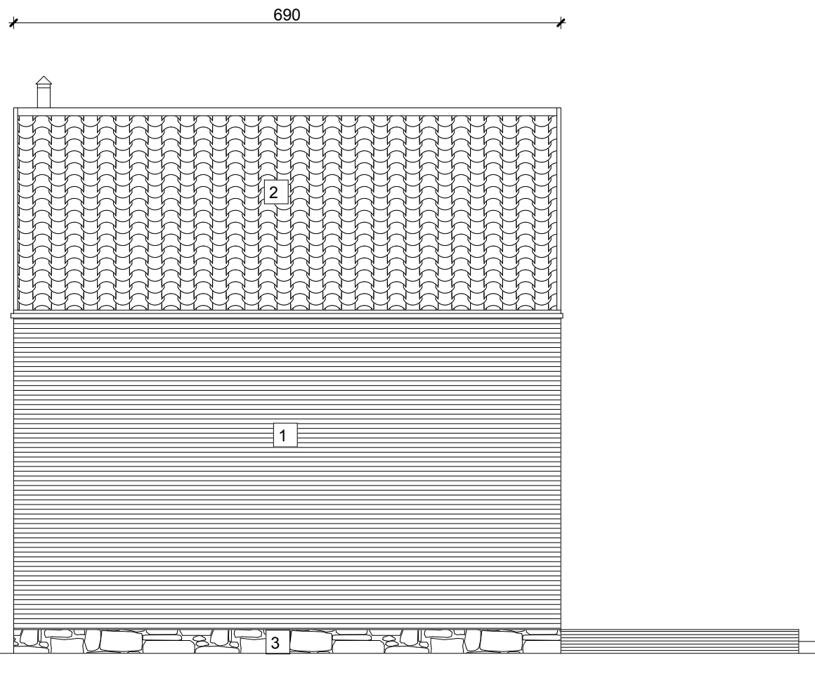
ELEWACJA LEWA
