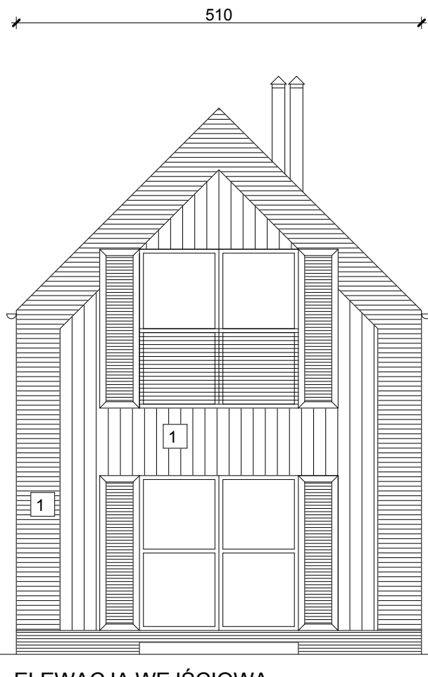
ELEWACJA WEJŚCIOWA
