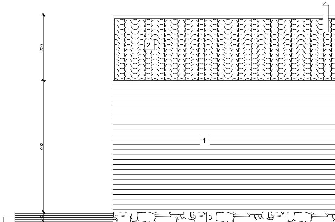
ELEWACJA PRAWA
