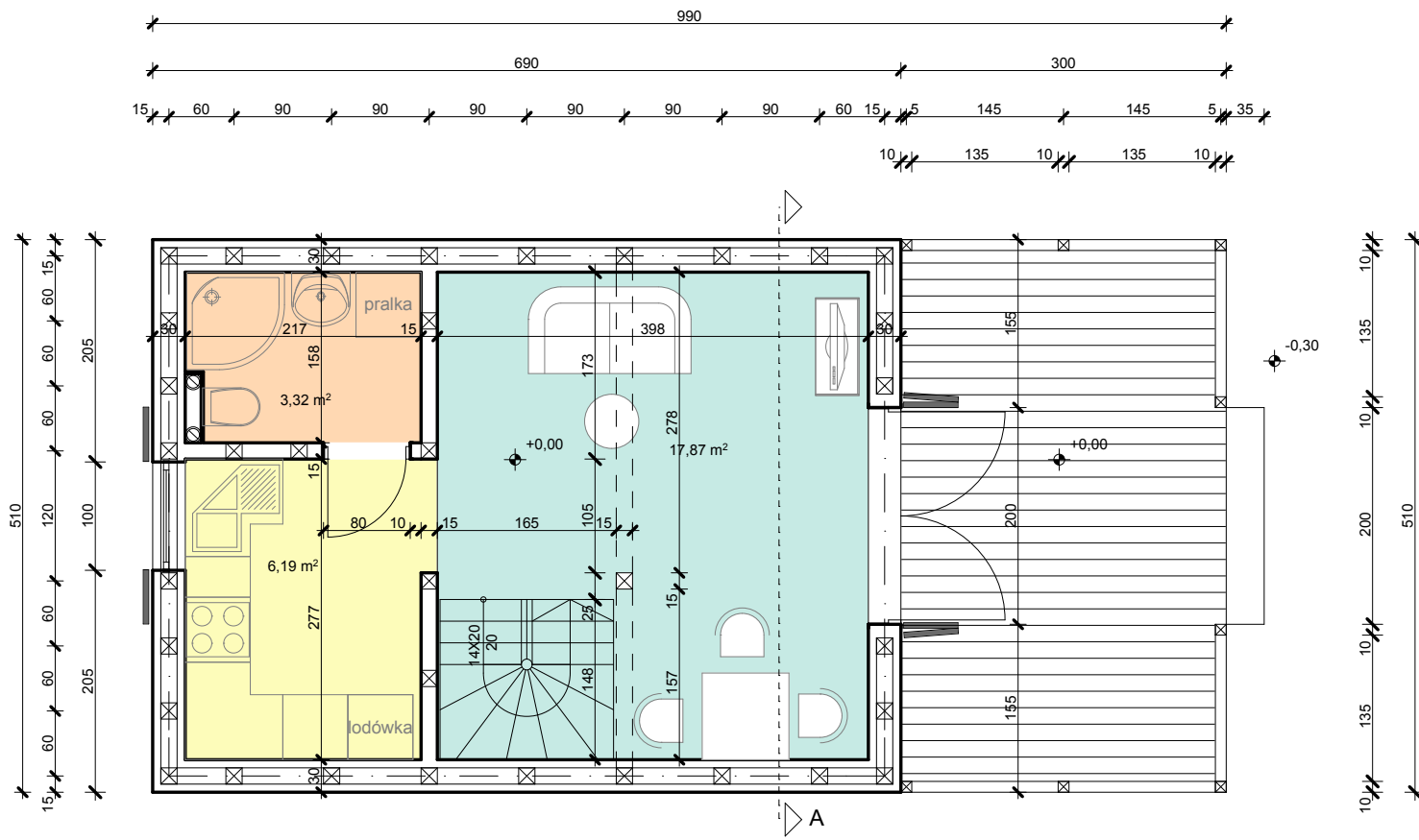
RZUT PARTERU PU = 27,38m 2
