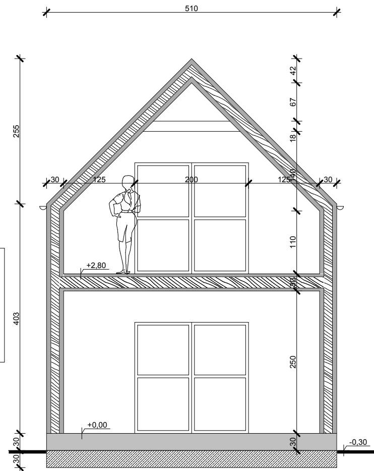
PRZEKRÓJ A-A
